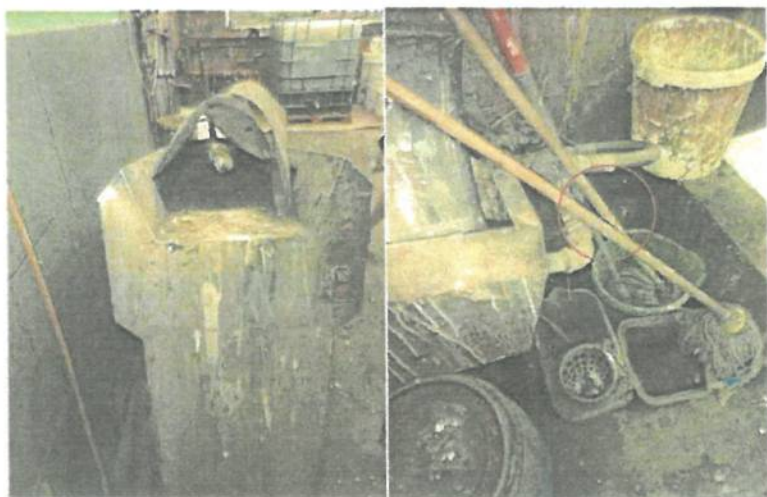
Fot. 6 i 7. Urządzenie wykorzystywane do mycia sit z maszyny STORK. Urządzenie posiada podłączenie do wody. Na zdjęciu czerwonym okręgiem zaznaczono odprowadzenie od maszyny, które zimuje się w ścianie.
